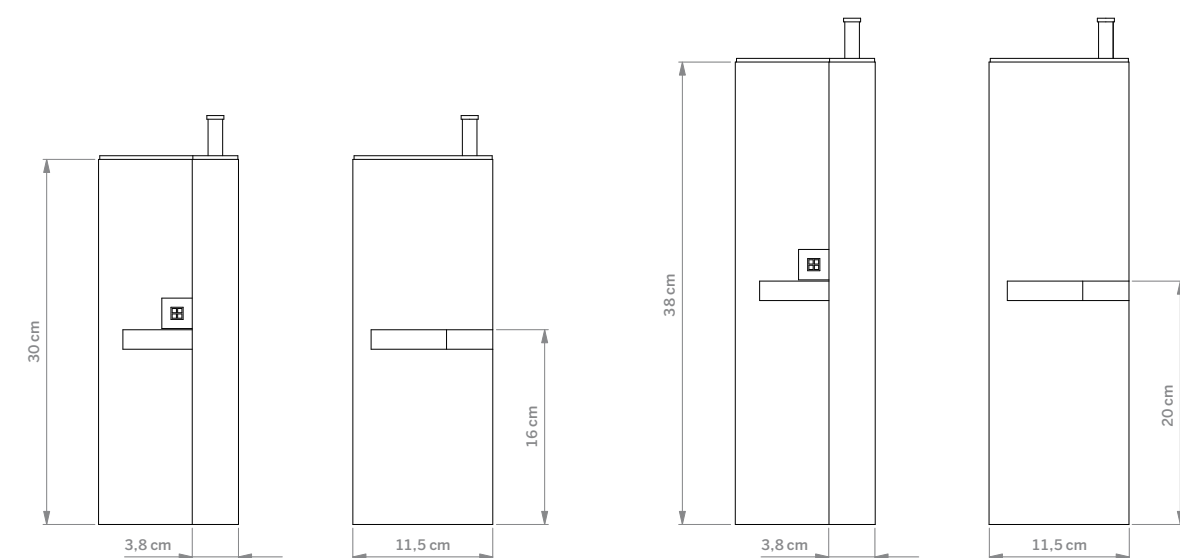
T57D Höhe verstellbar height adjustable hoogte verstelbaar 33–37 cm
